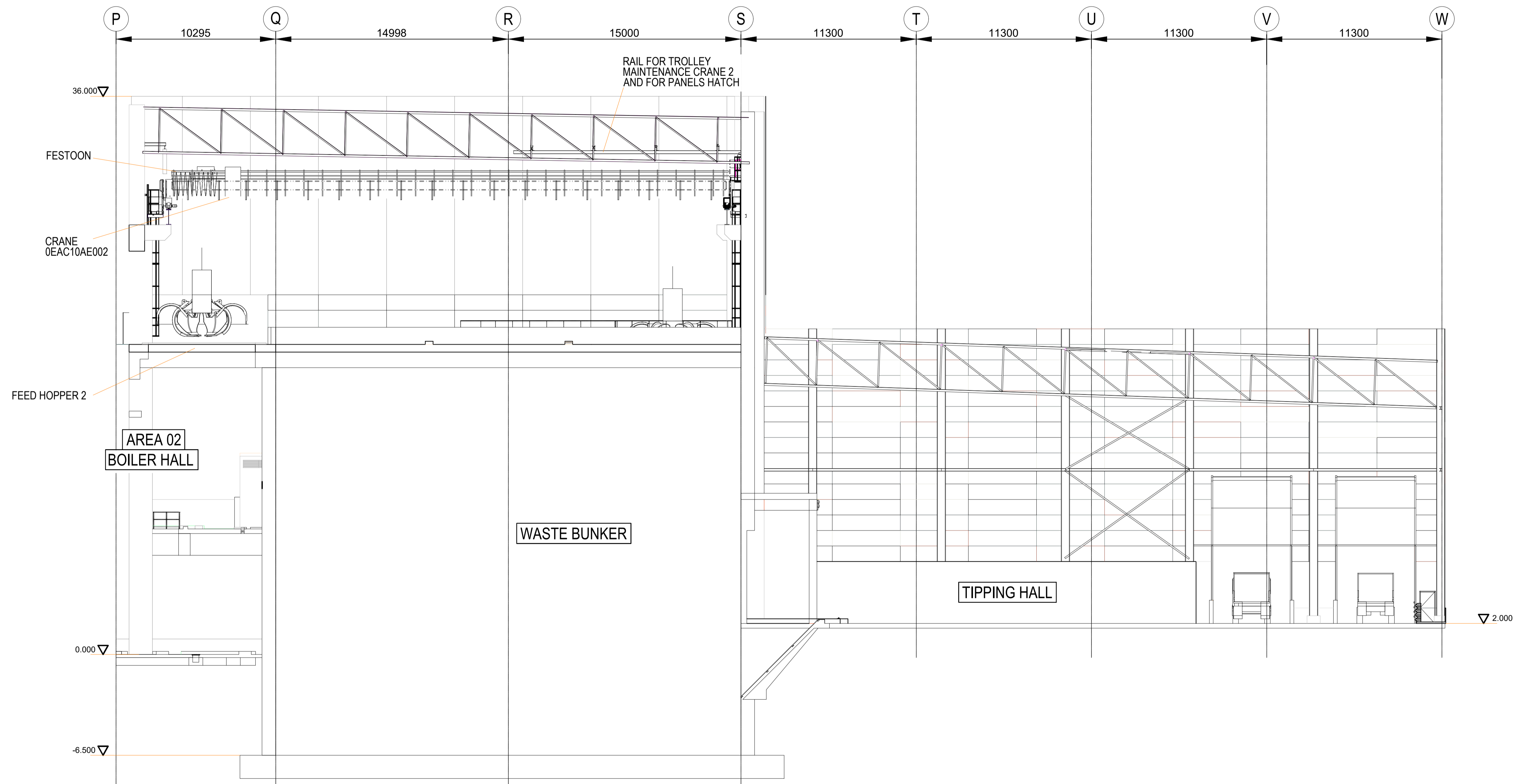
Section A-A Scale 1:150
